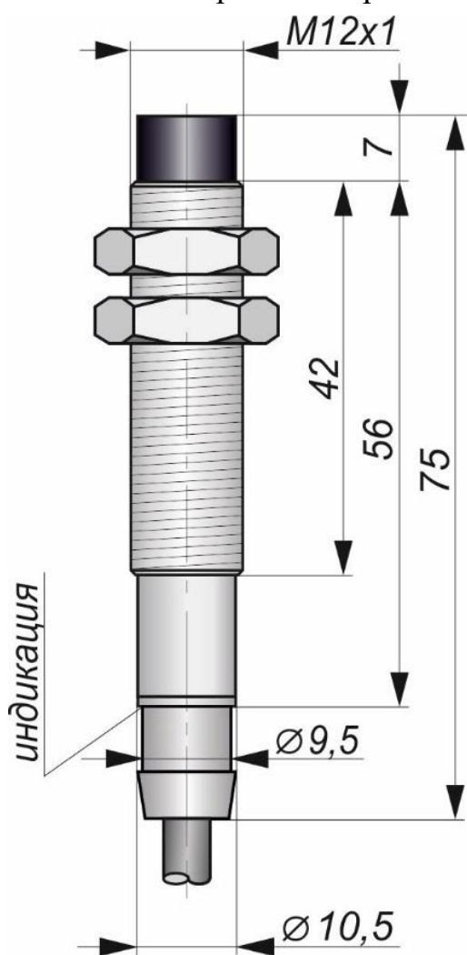
Габаритный чертеж
